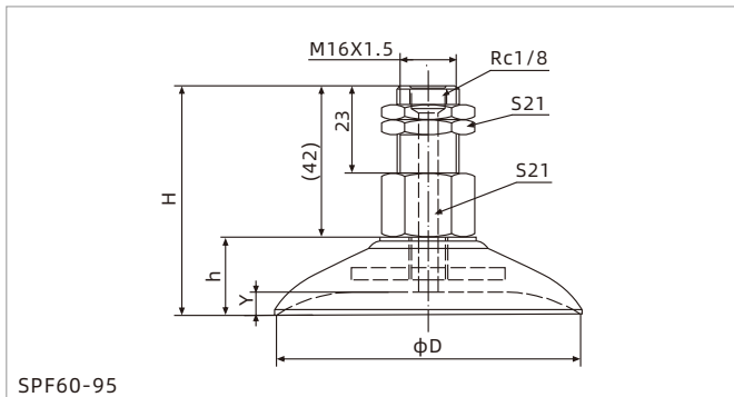
SPF60-95
