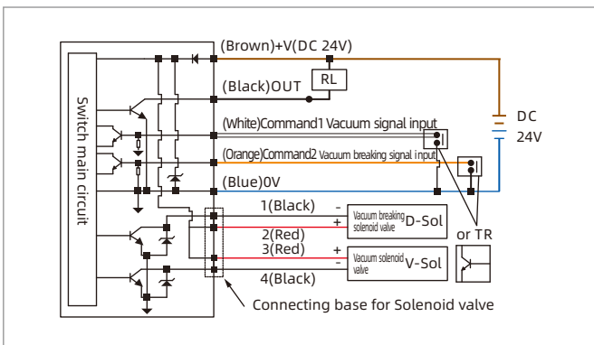
ZPDC-NE(NK/NEO)NPN output
