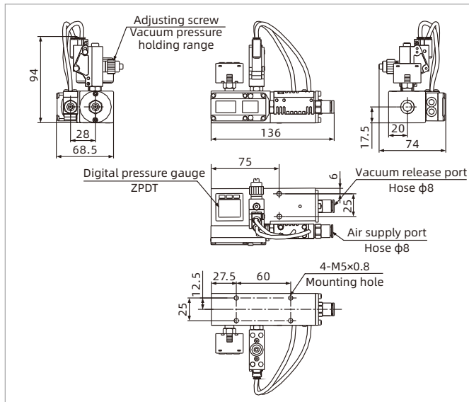
AZD20-ES
