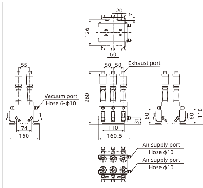
AZW-06V
