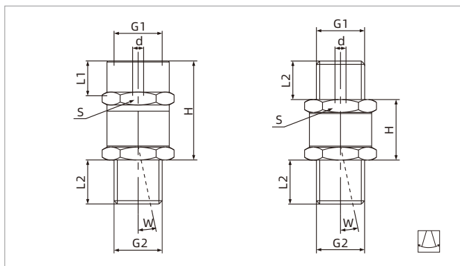
PJE-F-M
