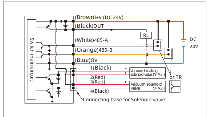
ZPDC-PR-E PNP output
