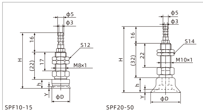
SPF10-15
