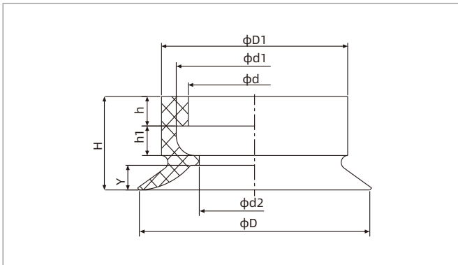
SPU10-25
