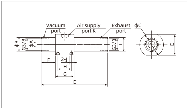
ACPF3-3
