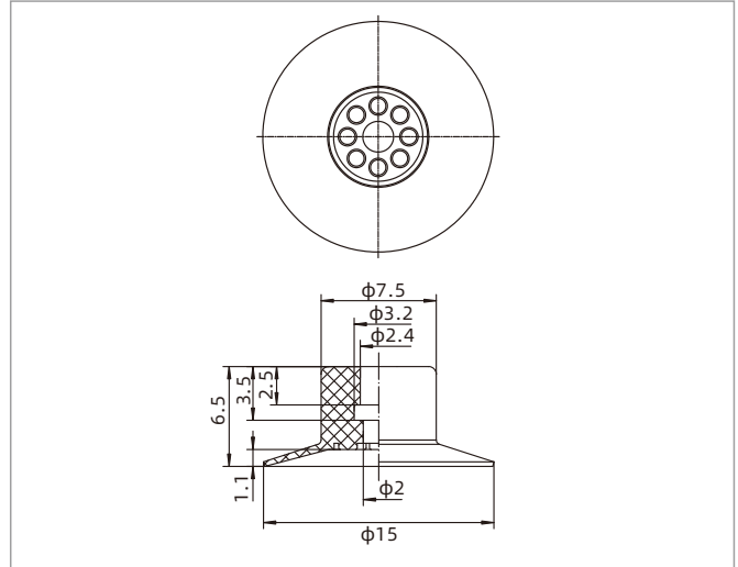
SPHMT15
