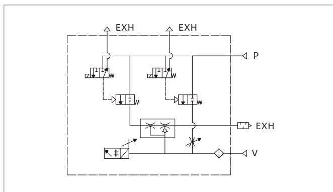
AZK-S(X/P/L)-N(P/NK/PK/NR/PR)
