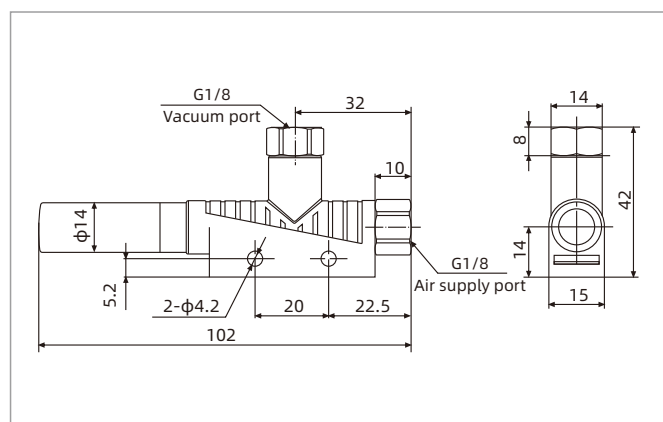
ASBP
