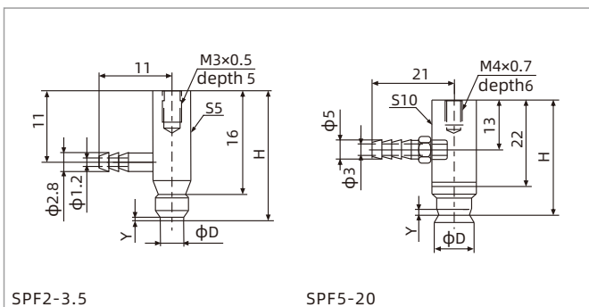
SPF2-3.5
