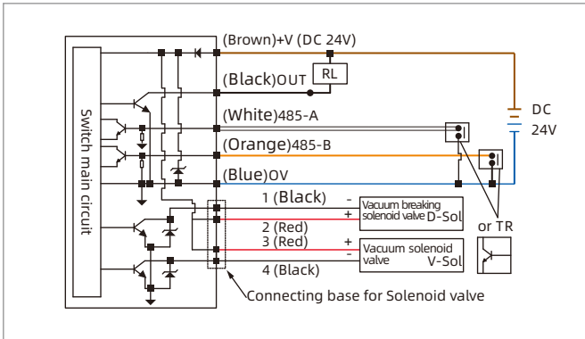
ZPDC-NR-E NPN output
