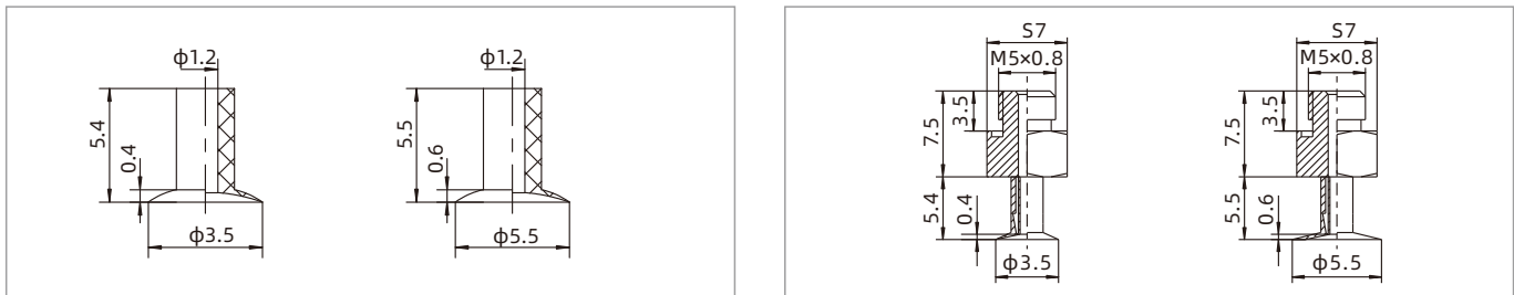
SUF3.5
