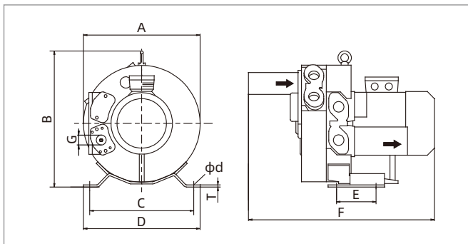
APB-420~620
