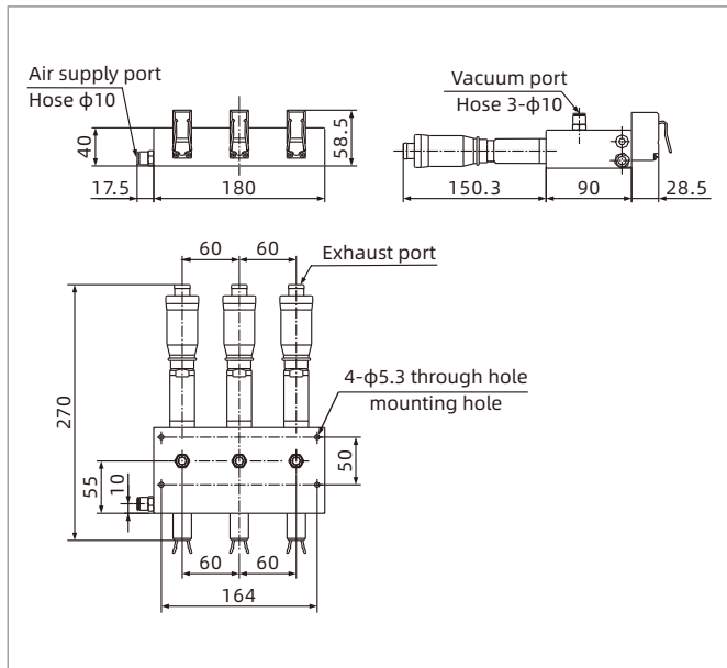
AZW-03V
