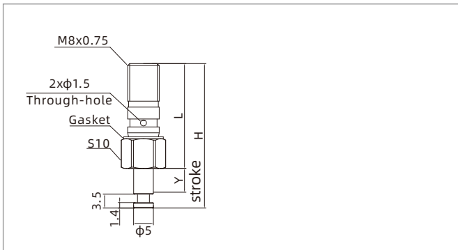
PPSP-I6D5-I8
