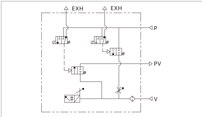
AZK-B-N(P)
